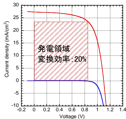
図：ペロブスカイト構造と、ペロブスカイト型太陽電池（変換効率20%）の特性
