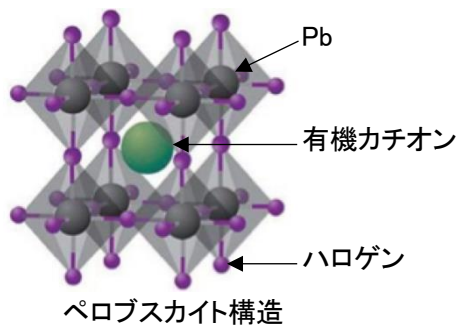
図：ペロブスカイト構造と、ペロブスカイト型太陽電池（変換効率20%）の特性
