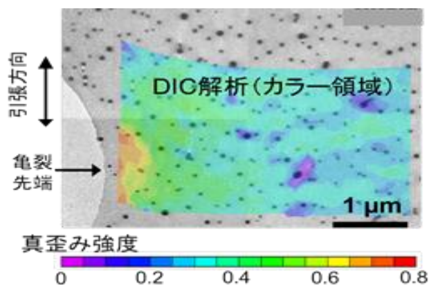
図：シリカ含有エポキシナノコンポジット薄膜の引張過程における透過型電子顕微鏡像と薄膜内歪み分布のデジタル画像相関（DIC）法による解析
