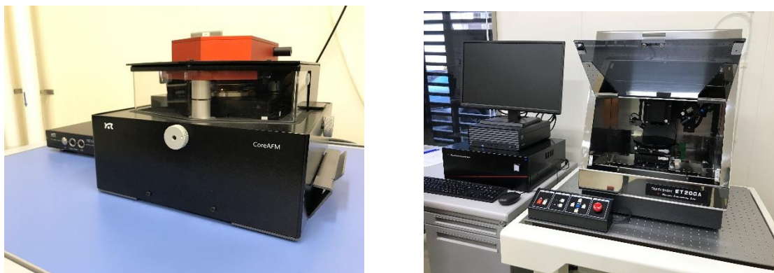
図：原子間力顕微鏡（左）と触針式表面あらさ計
