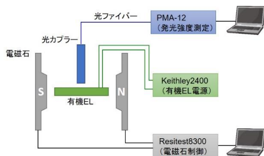
(a) 測定系の概略
