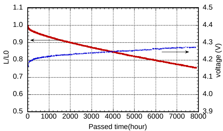
(e) 連続駆動寿命 ( 1000 \text{ cd}/\text{m}^2 スタート)
