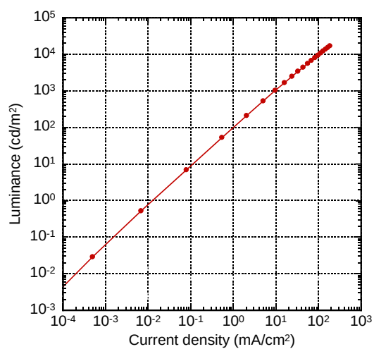
(b) L-J 特性
