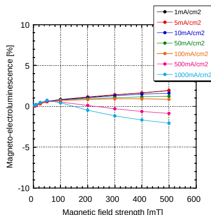
図 3-4. 発光強度の磁場依存性
