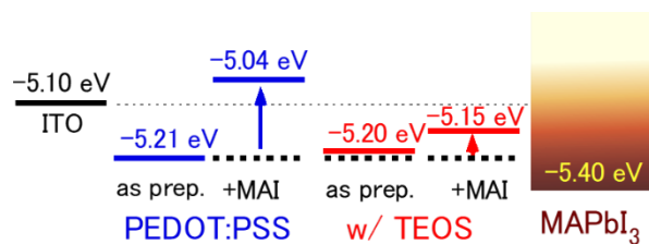
図3-9. TEOS添加によるエネルギーシフトの抑制
