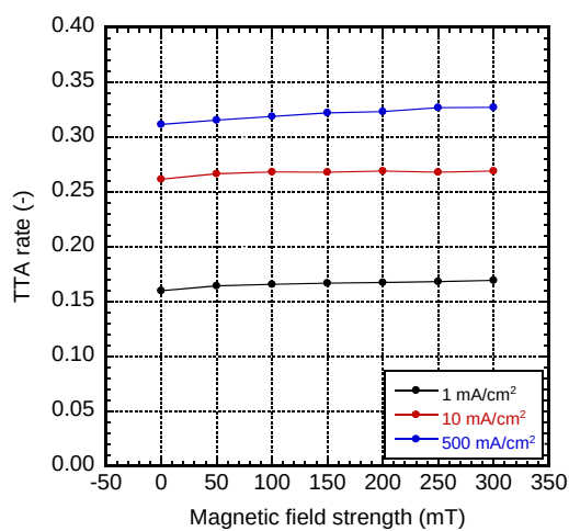
図 3-19 高性能青色有機 EL 素子の TTA 化率の磁場強度依存性
