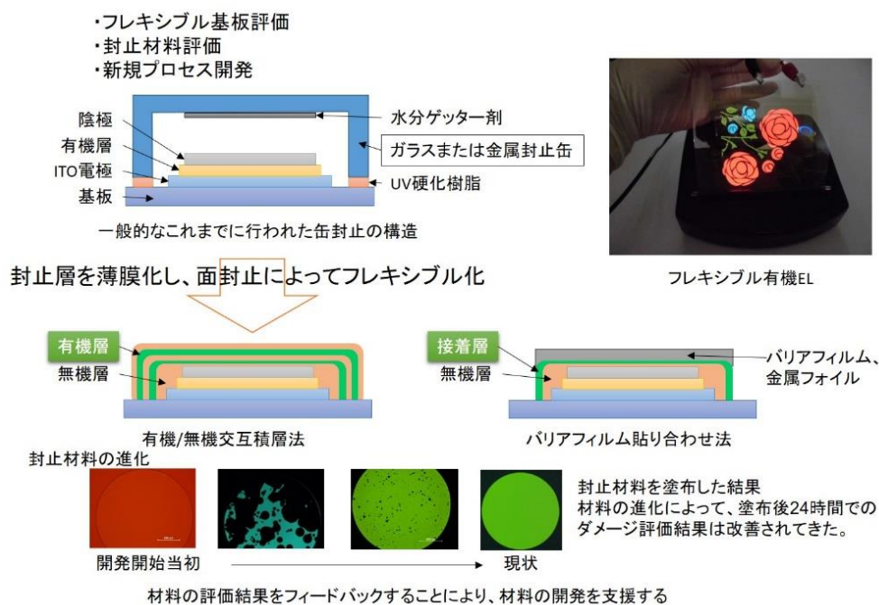
図 3-20 フレキシブル有機 EL を支える面封止技術（特に、有機層）の評価
