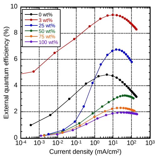
(c) EQE-J 特性
