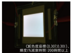
CIE色度座標(0.307,0.301)、輝度1%減衰時間>200時間以上 黄色発光TADF材料と既存の青色材料を用いたタンデム型白色有機ELデバイス
